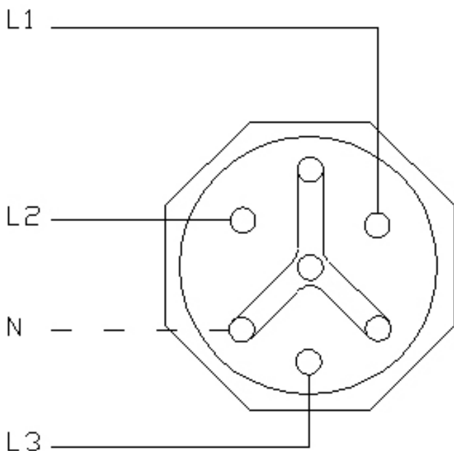
TÄHTIKYTKENTÄ PIENET TEHOT
